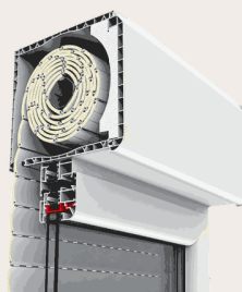
Caja aislada y eje de lamas
